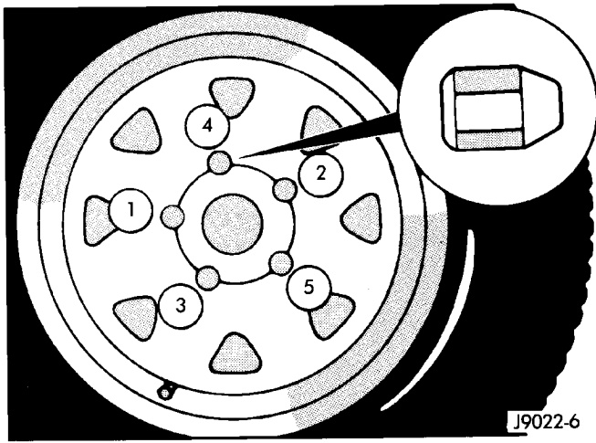
Fig. 5 Lug Nut Tightening Pattern
